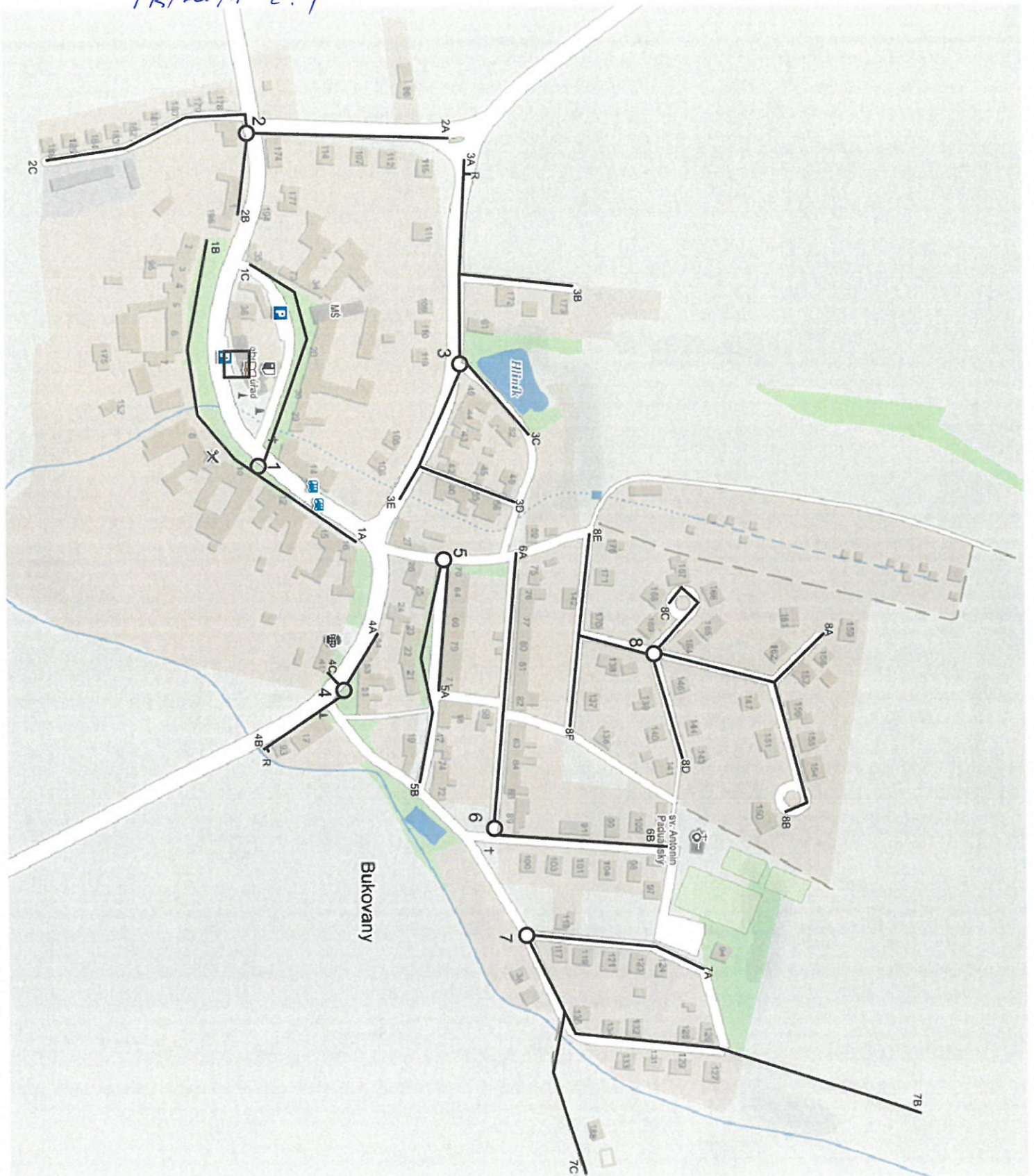
Obr. 1 - svazky mikrotubiček HDPE 7/3.5mm od rozvaděčů ke klientům - 1.6.2020
